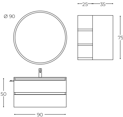
L 90 H 50 P 46
