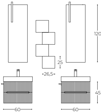
L 60 H 45 P 46
