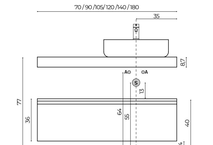
QUOTE PER TOP SCATOLARI CON BASI H.36 QUOTAS DISCHARGES FOR BOX-SHAPED WITH BASE UNIT H. 36
